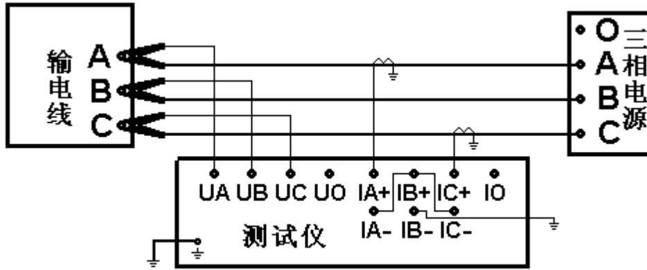
图3 三相三线外接电流互感器接线图
